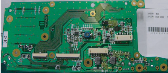
05P0844 (PANEL)
